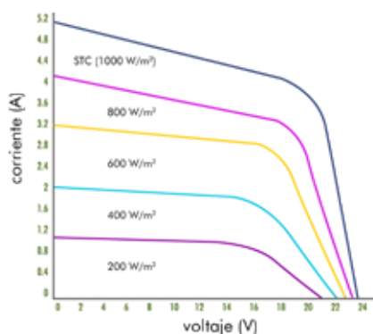
Curva IV a vari livelli di irraggiamento in condizioni di massa d'aria di 1.5 e temperatura celle di 25°C
