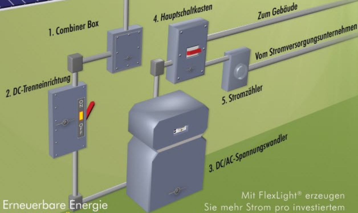
Kabelorganisationssystem
